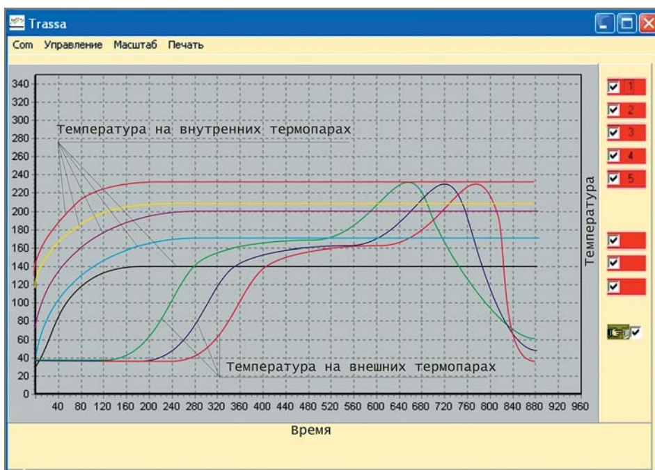
Рис. 7. График изменения температур снятый при пайке на установке инфракрасно-конвекционной пайки печатных узлов «S.M.D.-Трасса-5610»
